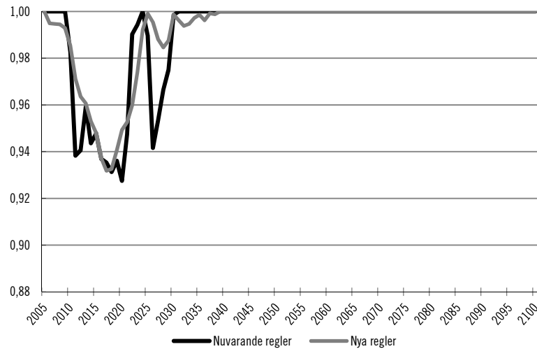
Figur 7.4 Ackumulerad balansering
