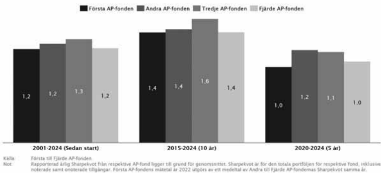
Figur 17: Första till Fjärde AP-fondens genomsnittliga Sharpekvot, 2001-2024
