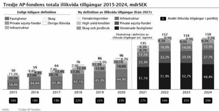
Figur 52: Tredje AP-fondens totala illikvida tillgångar, 2015–2024
