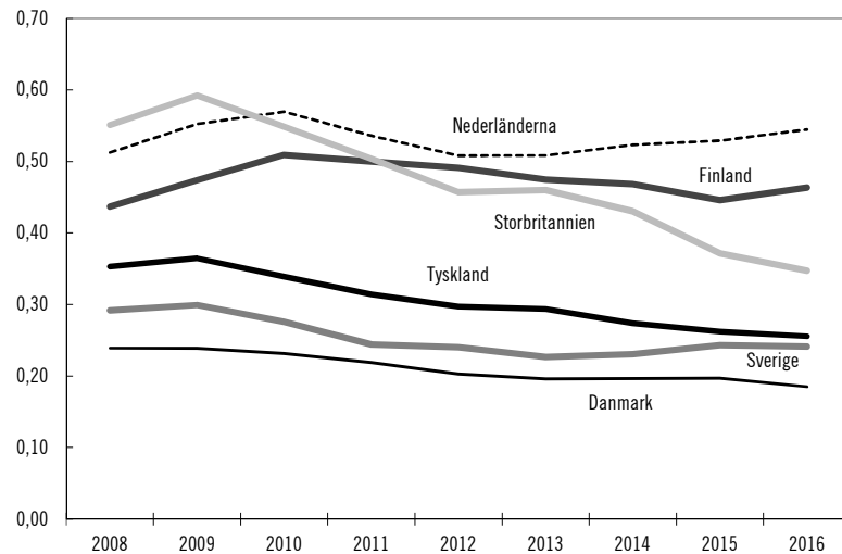
Figur 2.6 Utsläppsintensitet, kg/euro
